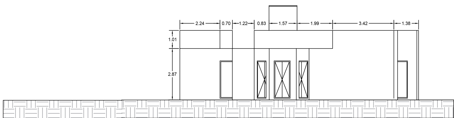
Elevation 1:100
